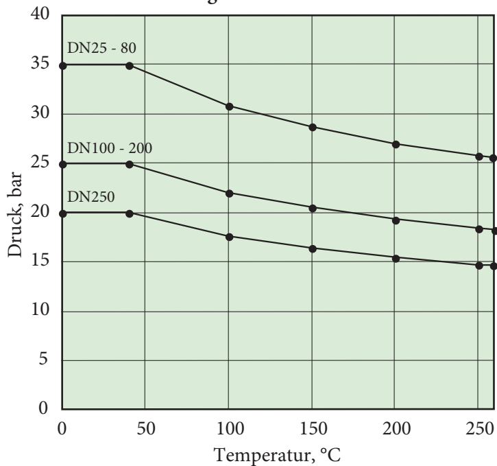
Max Betriebs-Differenzdruck im Regelbetrieb, RA Öffnungsbereich 70 % - 100 %
