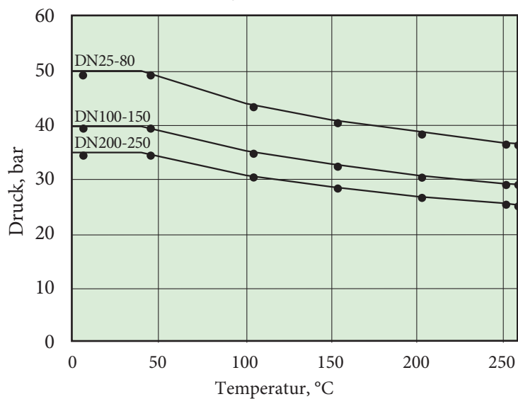
Max Betriebs-Differenzdruck im Regelbetrieb, RA Öffnungsbereich 0 % - 70 %
