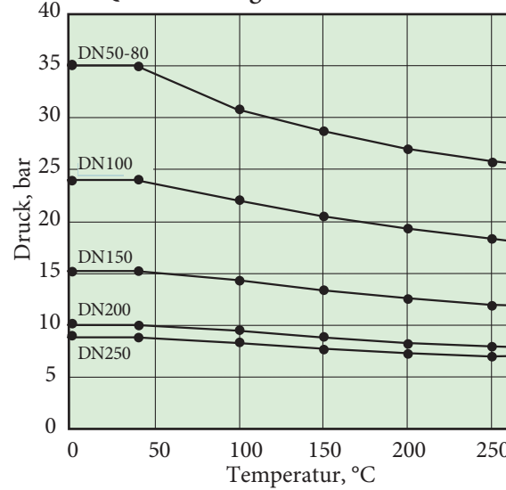
Max Betriebs-Differenzdruck im Regelbetrieb, Q-RA Öffnungsbereich 60 % - 100 %
