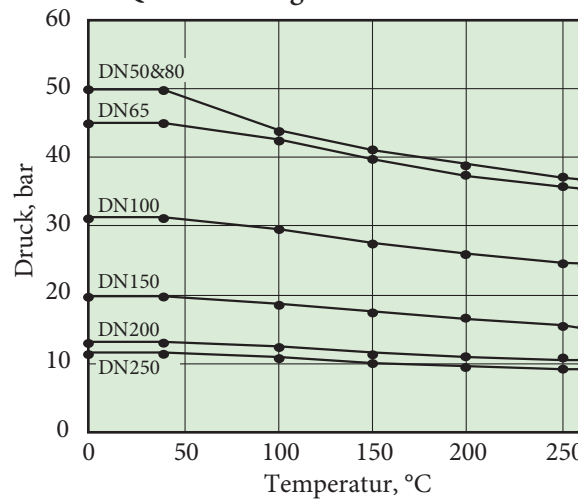
Max Betriebs-Differenzdruck im Regelbetrieb, Q-RA Öffnungsbereich 60 % - 100 %
