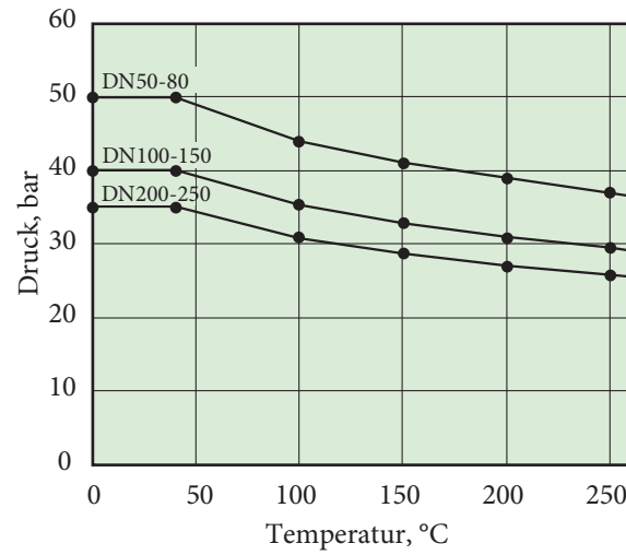
Max Betriebs-Differenzdruck im Regelbetrieb, Q-RA Öffnungsbereich 30 % - 60 %
